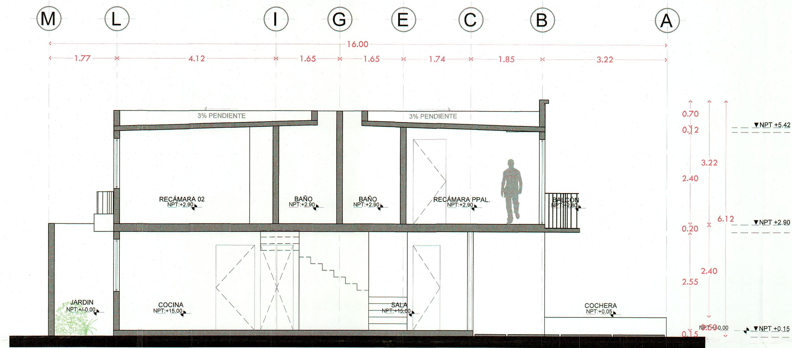
Corte B-B' arquitectónico
