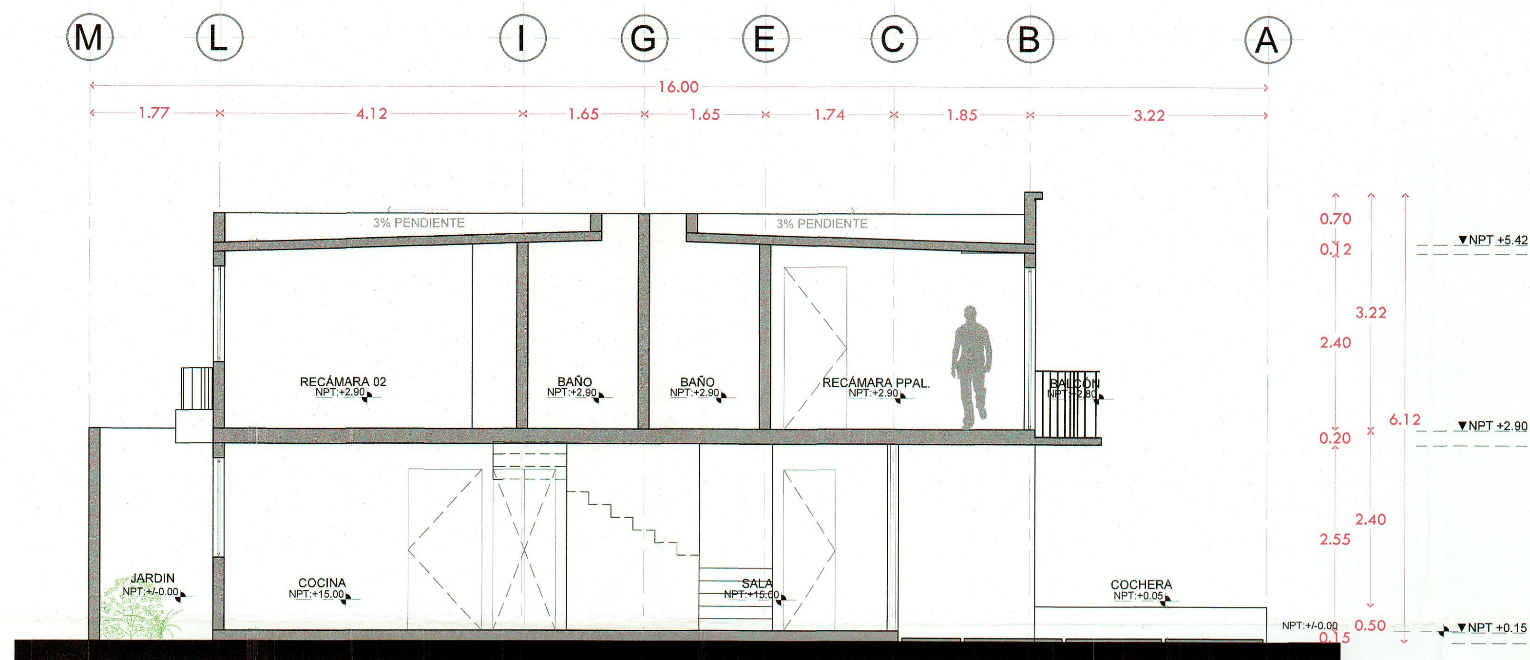
Corte B-B' arquitectónico
