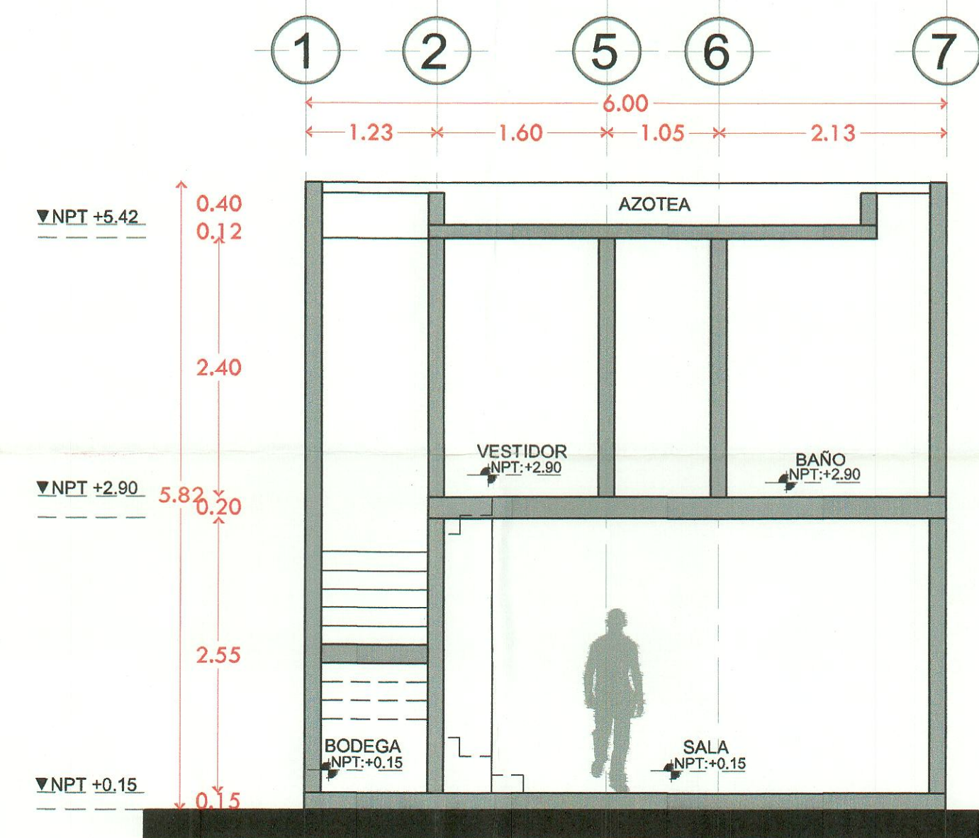
Corte A-A' arquitectónico
